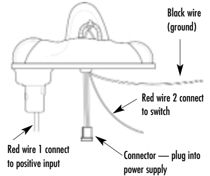
Wiring
