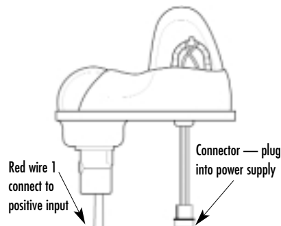
Wiring
